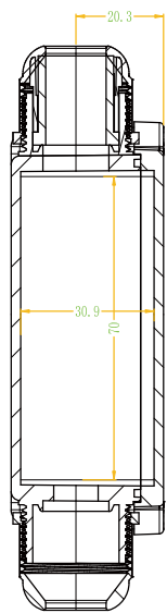
SECTION A-A
